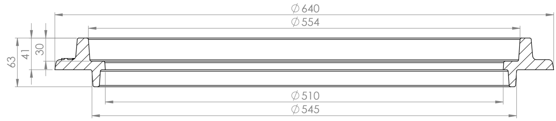
SECTION A-A
