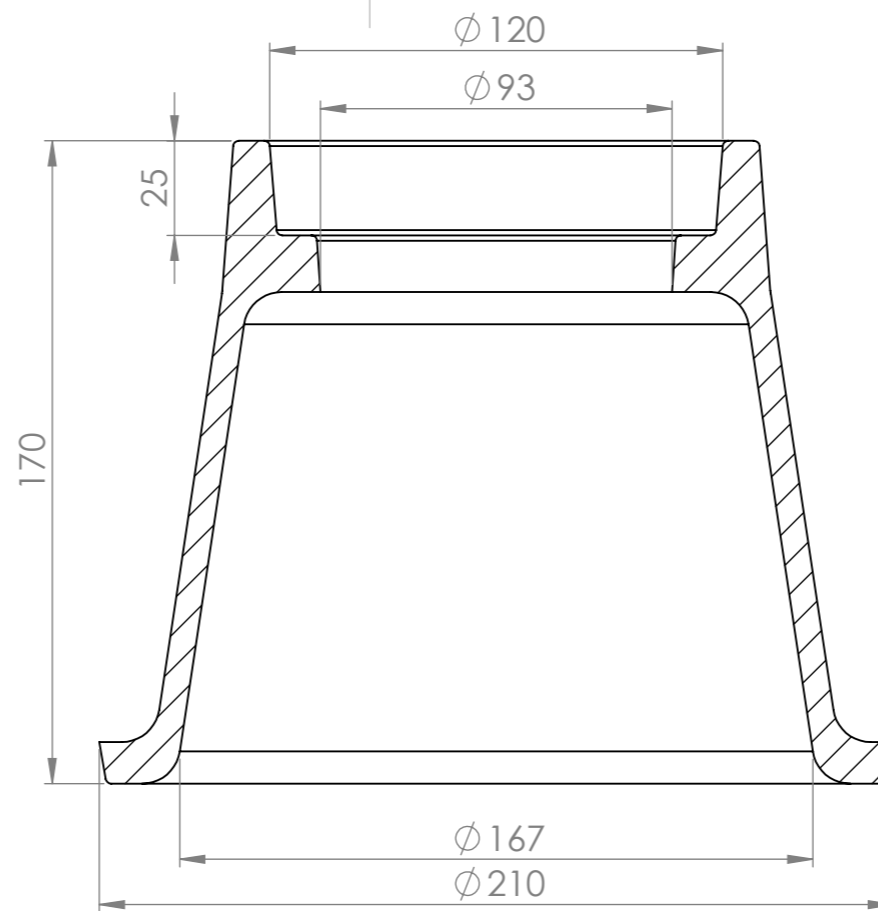
SECTION A-A
