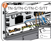
7 AC and equipotential bonding scheme
