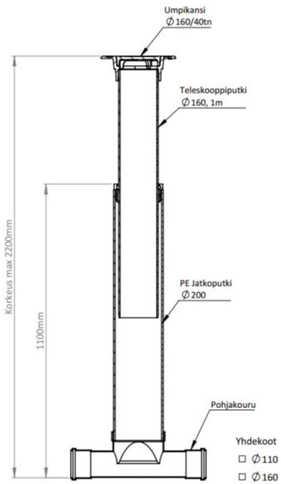
SECTION A-A
