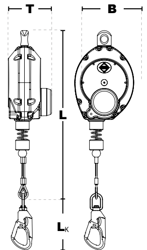
IKV 21 (EN 362:2004) with fall indicator
